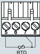
Трехпроводная система
