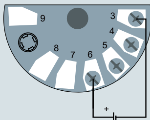
Вход напряжения (однополюсный или двухполюсный)
