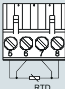
Четырехпроводная система
