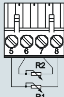
Формирование среднего значения / разности 1)
