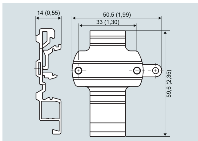
Переходник на DIN-рейку, размеры в мм (дюймах)
