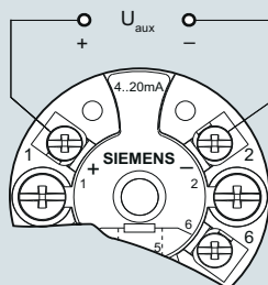
Подключение вспомогательного питания ( U_{аух} )
