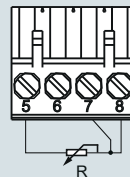
Трехпроводная система
