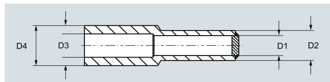
Габаритные размеры термогильз
