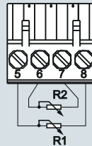
Формирование среднего значения / разности 1)
