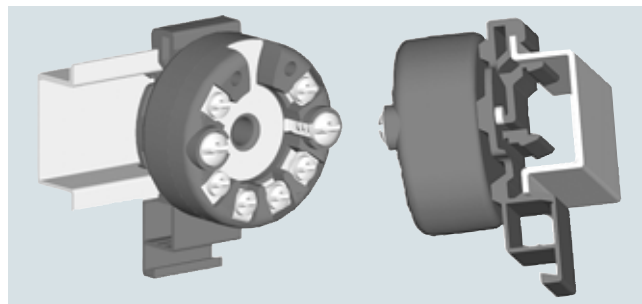
SITRANS TH200, монтаж измерительного преобразователя на DIN-рейку
