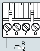
Двухпроводная система 1)
