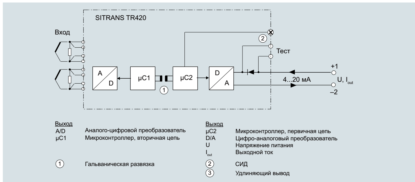
SITRANS TR420, функциональная блок-схема
