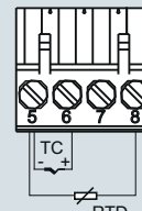
Компенсация холодного спая с внешним Pt100 в двухпроводной системе 1)
