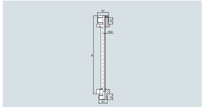
Удлинение (1, 2, 3), регулируемое, европейское, цилиндрическое, размеры в мм (дюймах)
