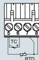
Компенсация холодного спая с внешним Pt100 в трехпроводной системе
