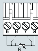
Четырехпроводная система
