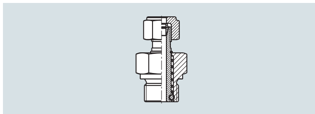
Подпружиненный компрессионный фитинг
