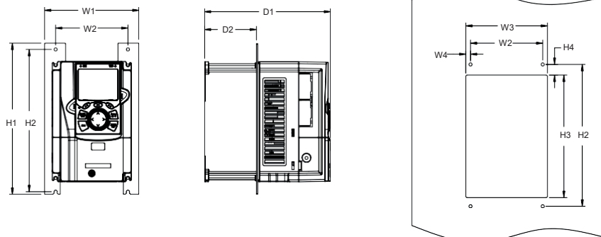
Рис 0.9 Схема фланцевого монтажа ПЧ напряжением 380 В, от 1,5 до 75 кВт
