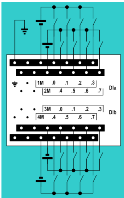
6ES7 221-1BH30-0XB0*
