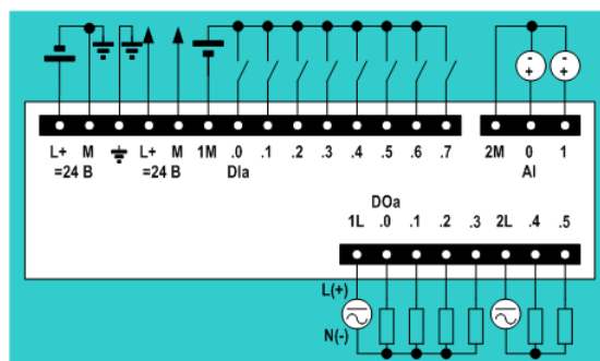
6ES7 212-1HD30-0XB0
