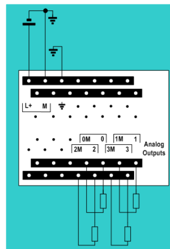
6ES7 232-4HD30-0XB0
