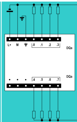
6ES7 222-1BF30-0XB0
