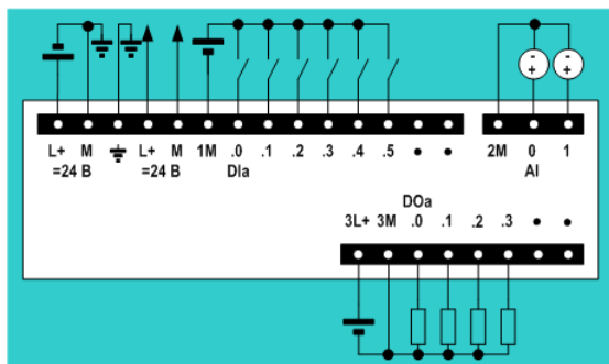
6ES7 211-1AD30-0XB0
