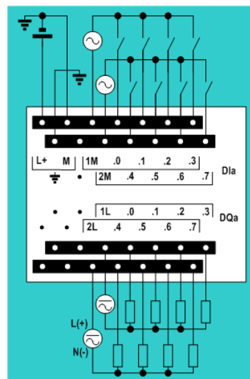
6ES7 223-1QH30-0XB0
