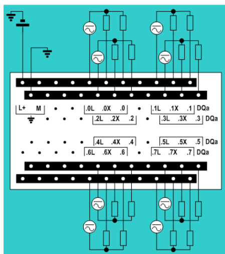
6ES7 222-1XF30-0XB0
