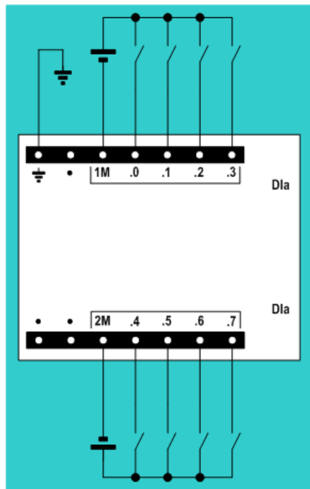
6ES7 221-1BF30-0XB0*
