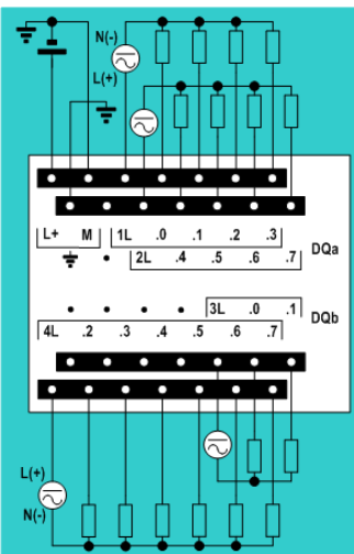
6ES7 222-1HH30-0XB0
