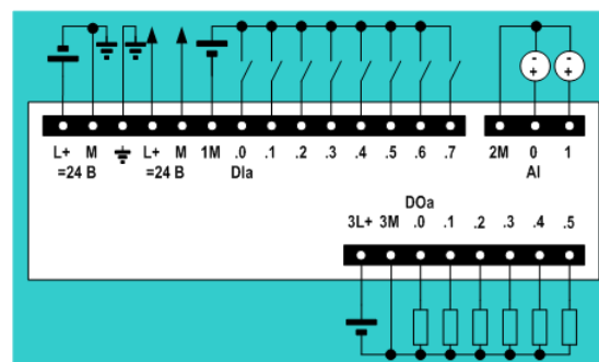
6ES7 212-1AD30-0XB0
