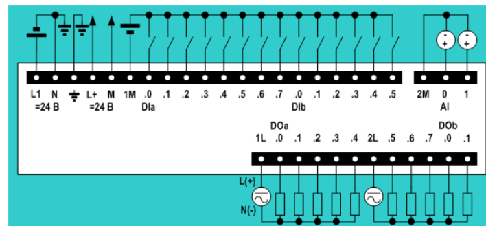
6ES7 214-1HE30-0XB0
