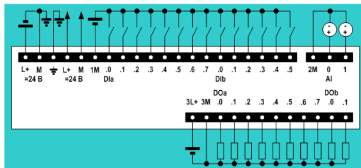
6ES7 214-1AE30-0XB0
