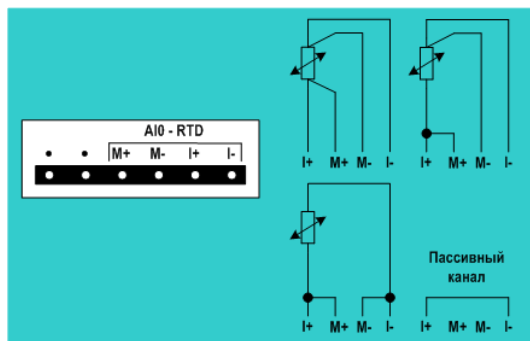
6ES7 231-5PD30-0XB0
