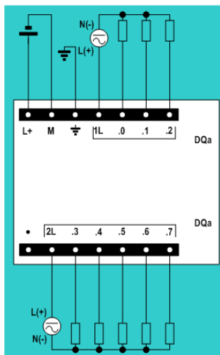
6ES7 222-1HF30-0XB0
