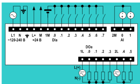
6ES7 212-1BD30-0XB0
