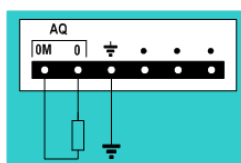
6ES7 232-4HA30-0XB0
