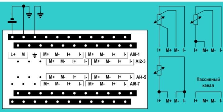
6ES7 231-5PF30-0XB0
